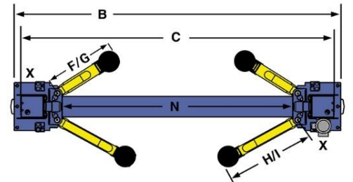
AVISO: Unidad de Energía puede colocarse en cualquiera de los puntos marcados por una X.
