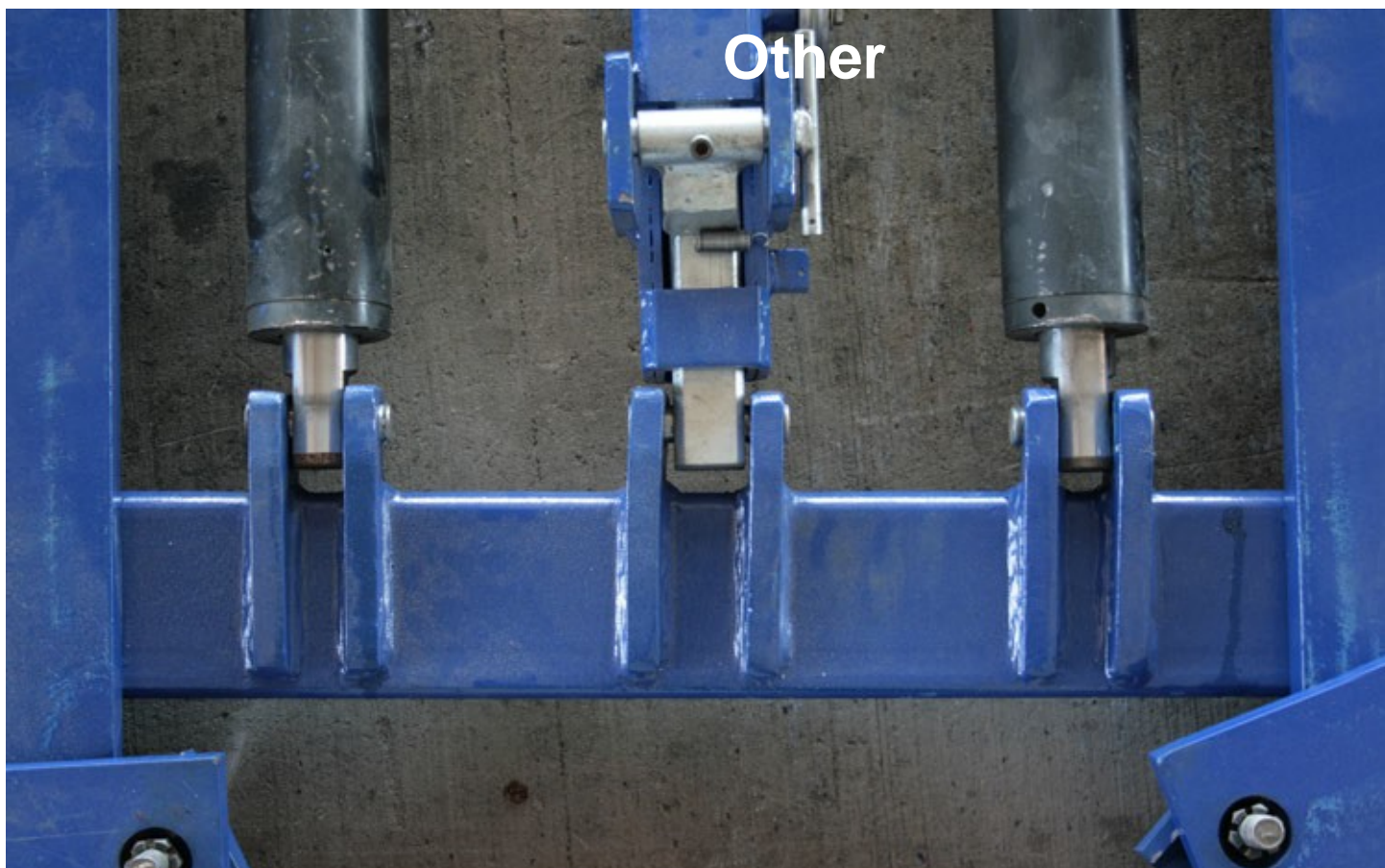
Marca Barata: Sistema de Sujeción del Cilindro
